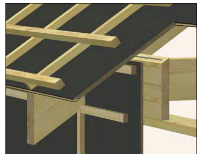
Overgang vegg/tak med sperreutstikk
